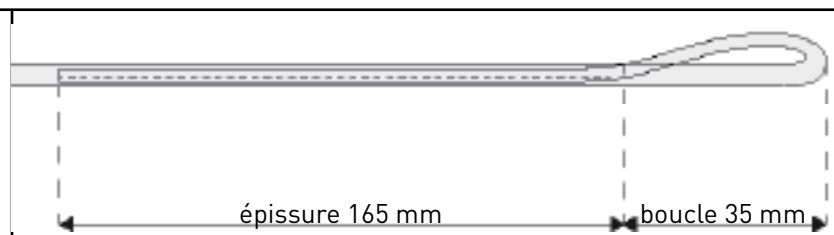
Schéma de principe du pod fourni :
