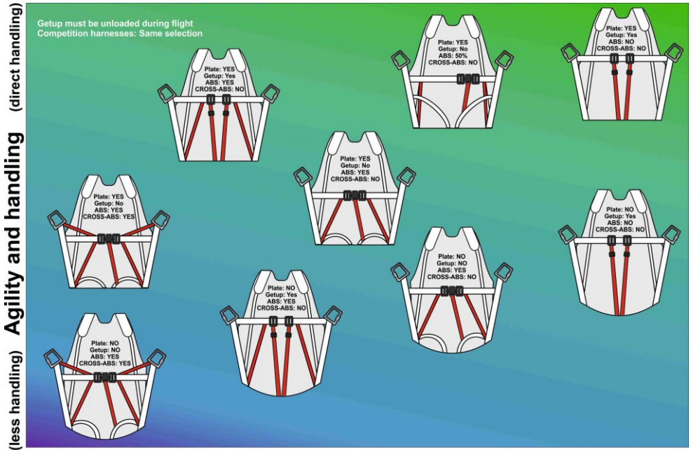
(very stable) Stability and damping (intensive communication) Abb. 4. Übersicht verschiedene Gurtzeuggeometrien und deren Dämpfung
