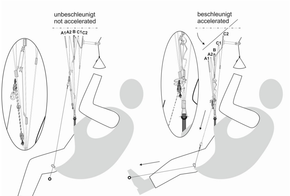
Funktionsweise Fußbeschleuniger HELIOS RS
