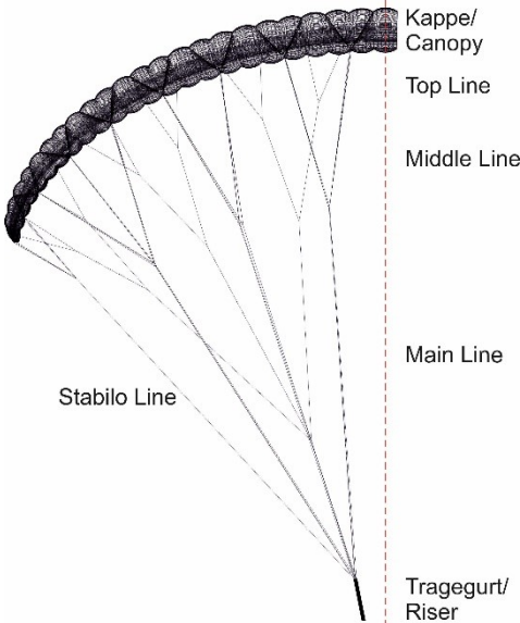
Gittermodell HELIOS RS
