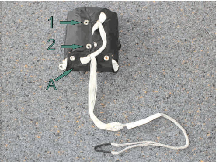
30b. Innencontainer mit den Fangleinen verschließen. Zuerst die lange Seite (Nr. 1). Nr. 2) wird zusammen mit der mittleren Öse des verbleibenden Containerlappens A geschlossen.
