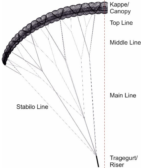
Abb. 1. Gittermodell ARCUS 2 RS
