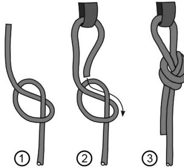
Abb. 4. Sackstich- Knoten
