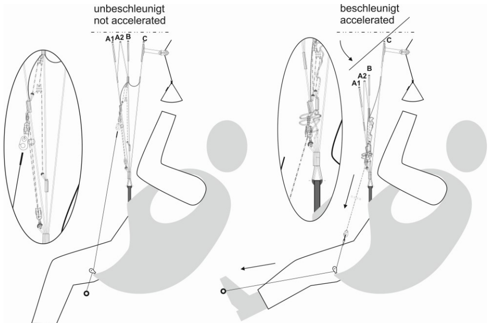
Abb. 7. Funktionsweise Fußbeschleuniger ARCUS 2 RS
